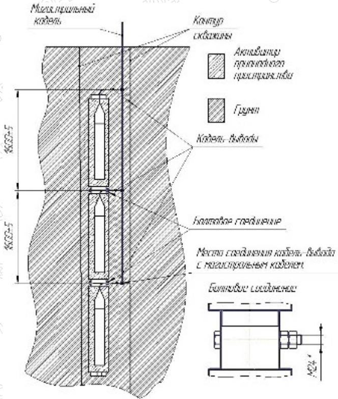
Установка АЗЖК-РА-ГУ в скважину с магистральным кабелем
