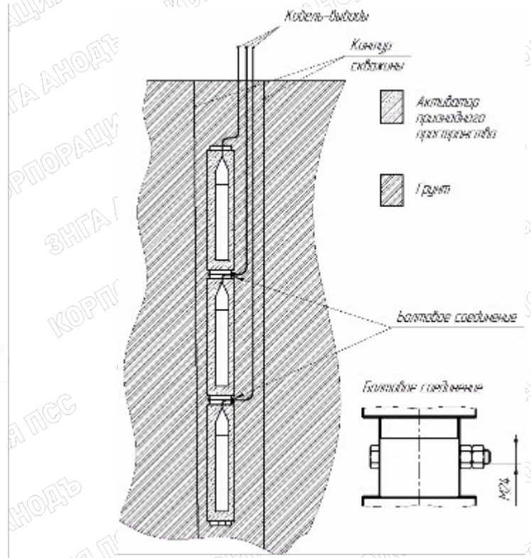
Установка АЗЖК-РА-ГУ в скважину без магистрального кабеля
